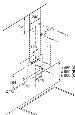
Wandinstallatie met luchtkanaal
