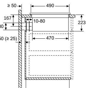
Zijaanzicht
