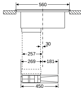
Vooraanzicht
