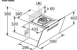
Apparaat in luchtcirculatiemodus zonder kanaal
