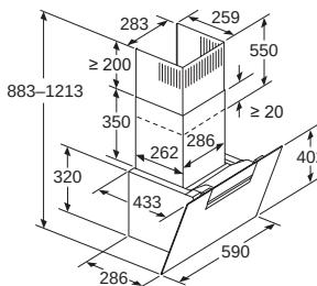
Apparaat in luchtcirculatiemodus
