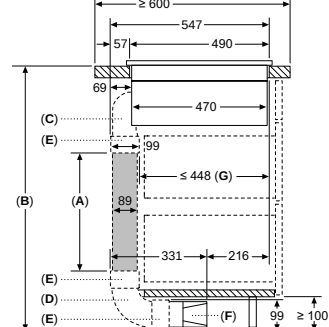
Zijaanzicht
