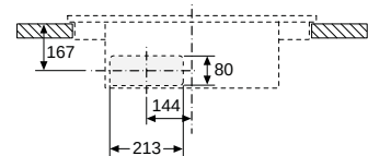
Vooraanzicht
