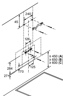
Afmeting in mm Wandinstallatie met luchtkanaal
