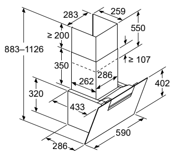
Afmeting in mm Apparaat in luchttafvoermodus
