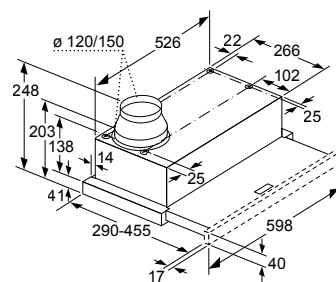
Diepteaanpassing van de filterafzuigkap tot 29 mm mogelijk Afmeting in mm
