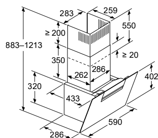
Afmeting in mm Apparaat in luchtcirculatiemodus
